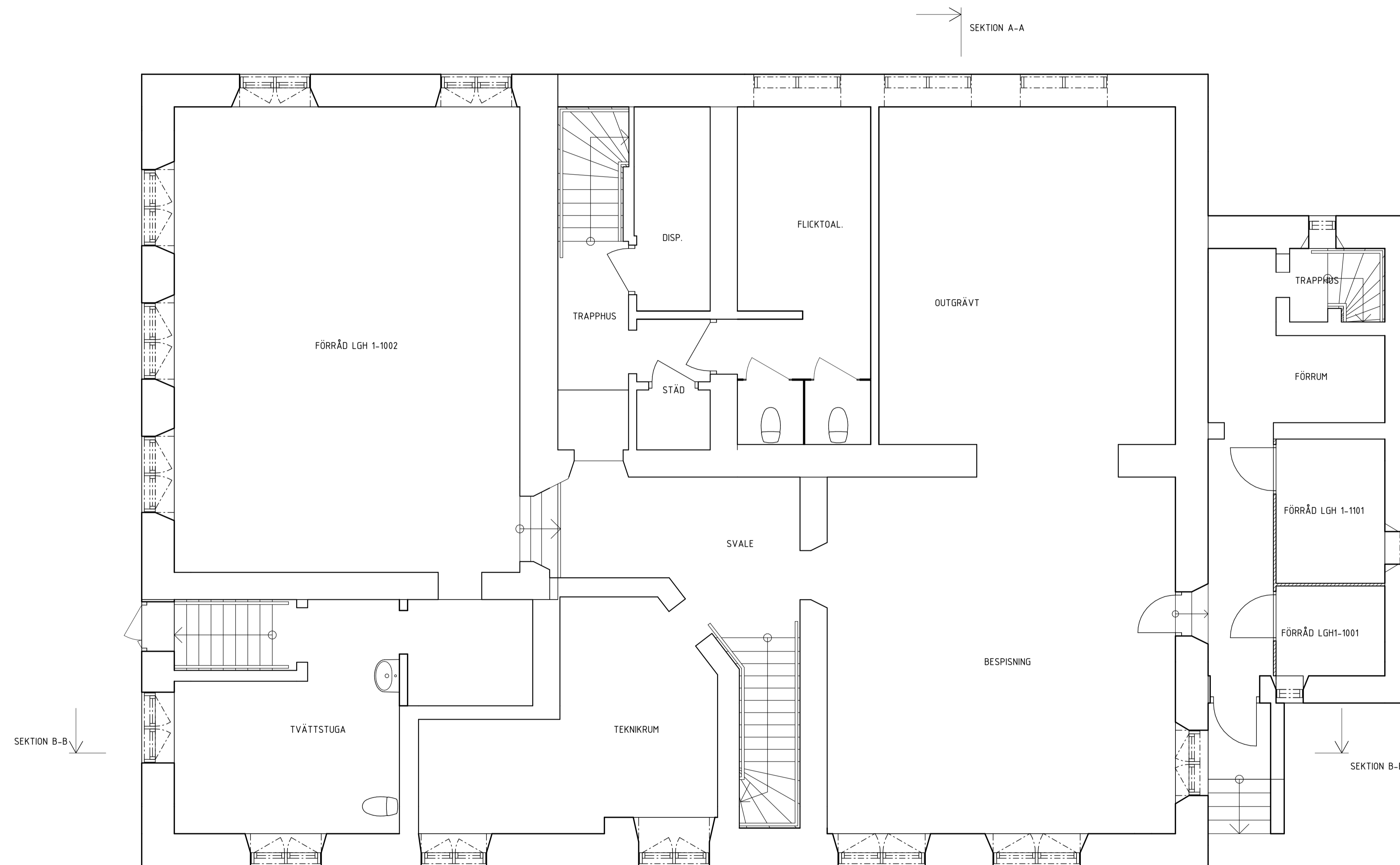
KÄLLARPLAN - NYTT 1 : 50
