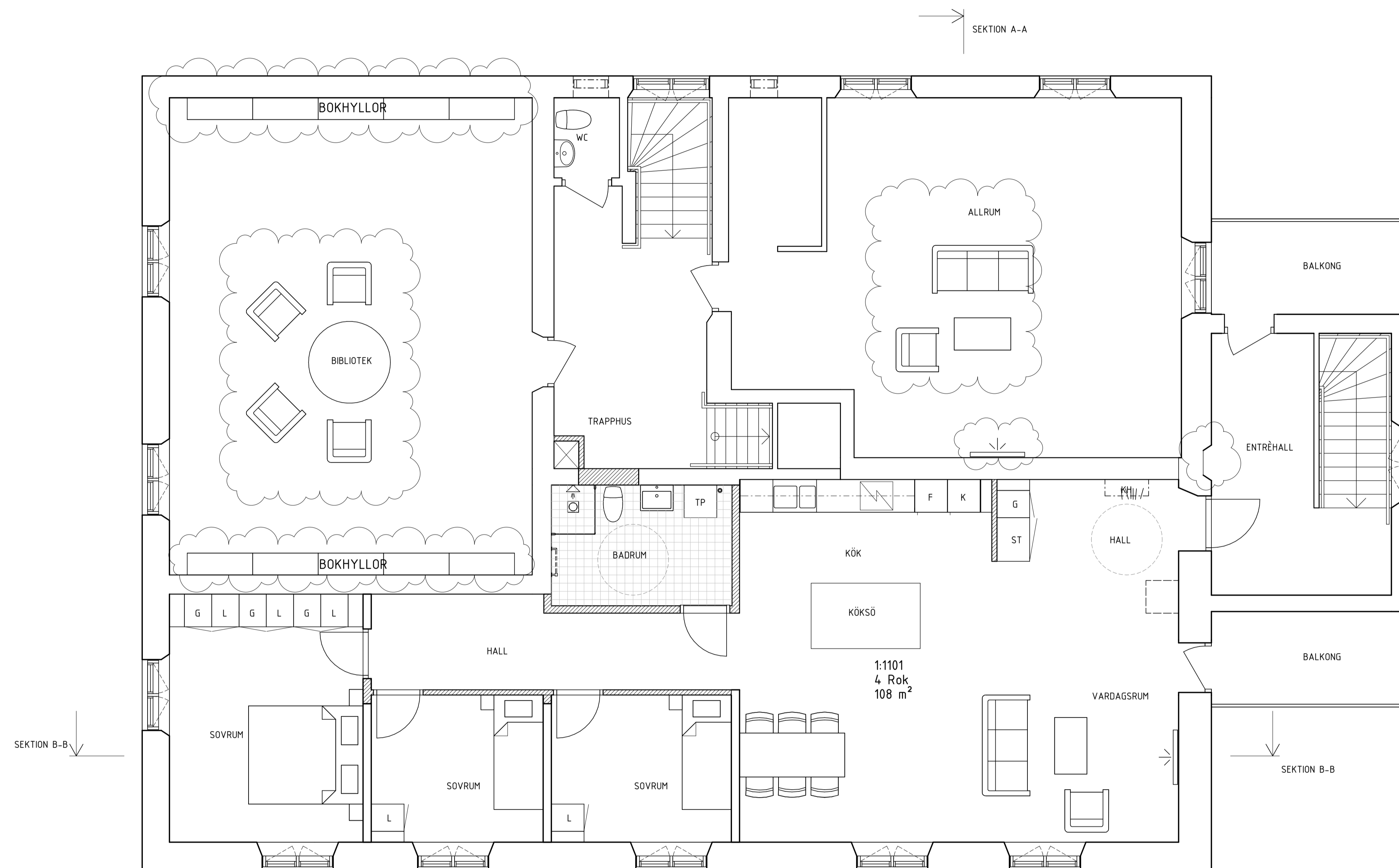
PLAN 2 - NYTT 1 : 50
